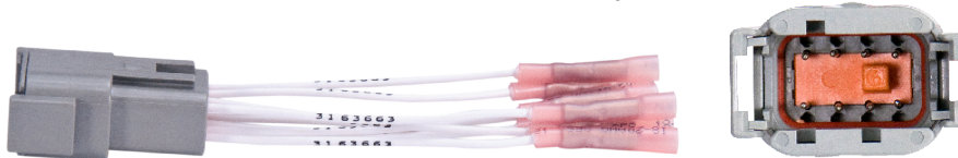
3163663 Deutsch™ 8 Position, DTM Series, Receptacle
